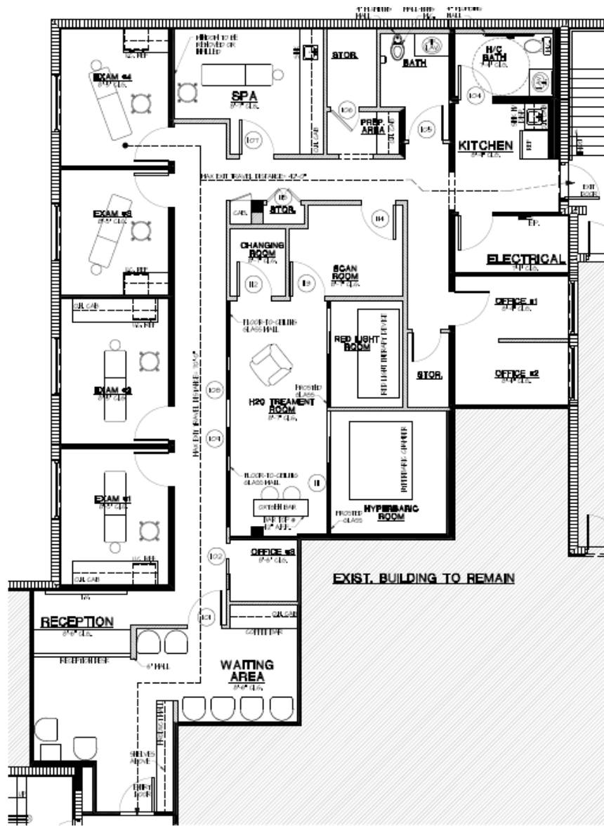
NOTE PLAN SCALE: 1/4" = 1'-0"
